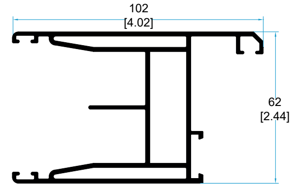
10505 HOJA PERIMETRAL.
