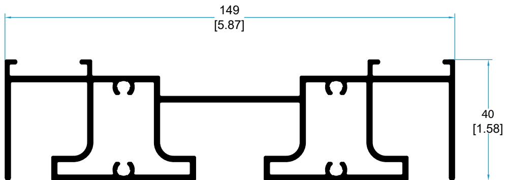
10502 CERCO SUPERIOR.
