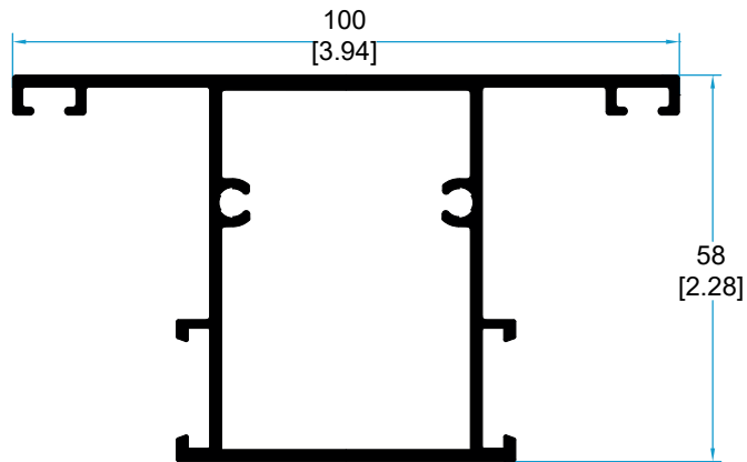
10509 PILASTRA.
