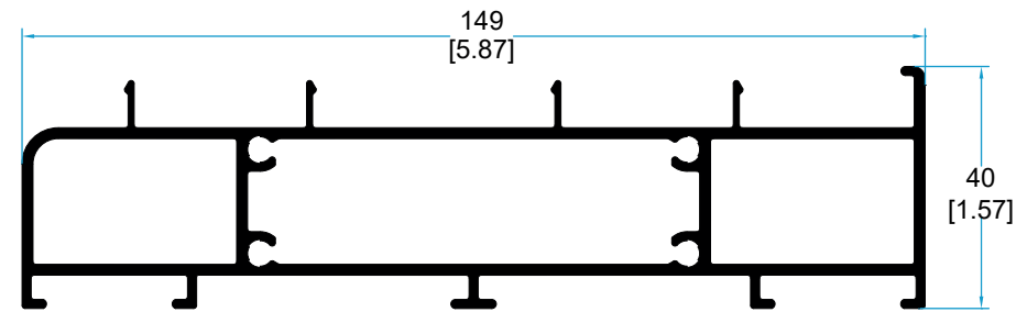
10501 CERCO INFERIOR.
