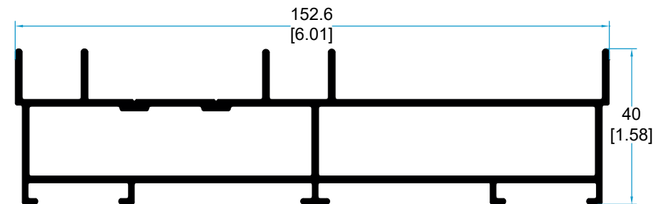
10508 CERCO LATERAL.
