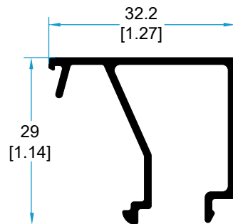
10530 JUNQUILLO ANCHO.
