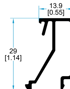
64263 JUNQUILLO 33 MM
