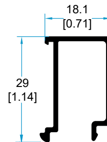
10531 JUNQUILLO ESTRECHO.
