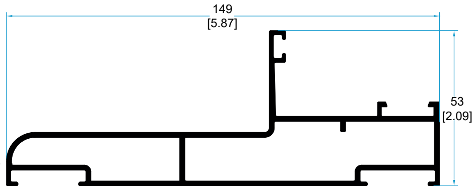
10503 FIJO PERIMETRAL.
