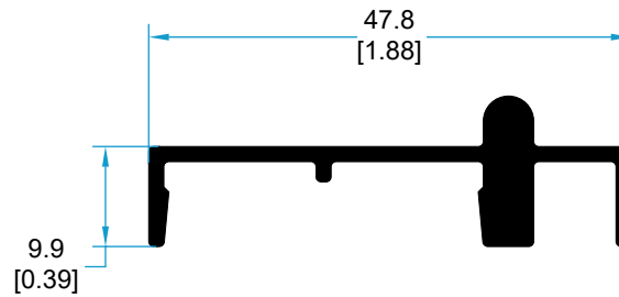
10511 RIEL RODADURA.
